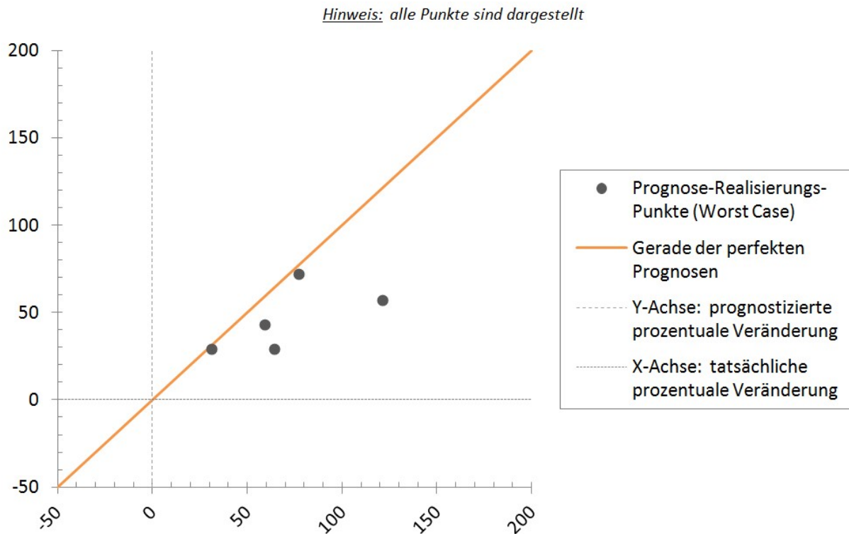
Abbildung 3.32: Prognose-Realisierungs-Diagramm mit Worst-Case-Prognosen 83
